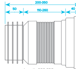
Mini Flexible Pan Connector
